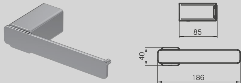
FR167/J5 Portarrollo. CR - FB
